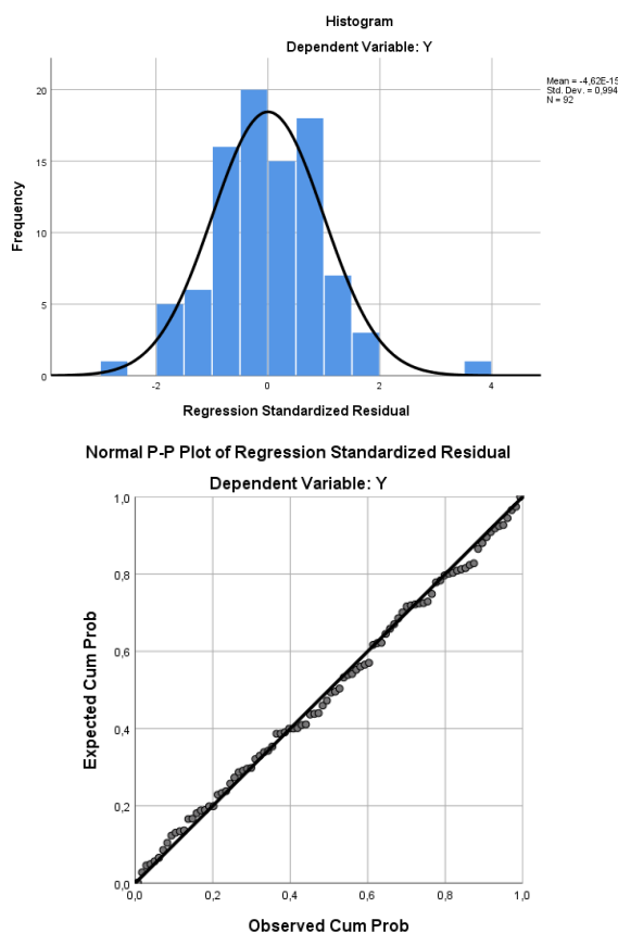
Gambar 1. P-P Plot of regression variabel komunikasi keluarga (X) terhadap variabel karakter santun (Y)
